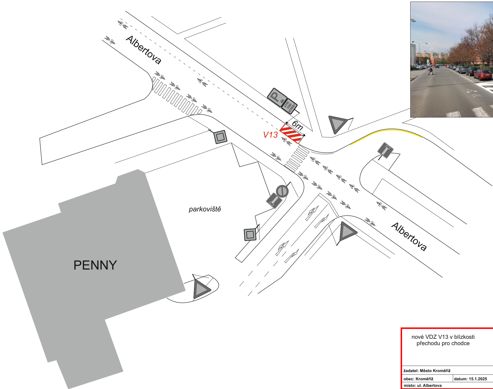
detail provedení VDZ
